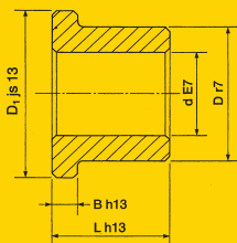
RUNDBOCKADE RADIALLAGER BRM 10 / BRM 80 INBYGGNAD (Gäller även flänslager)
